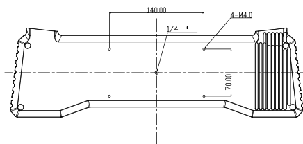
底视图
