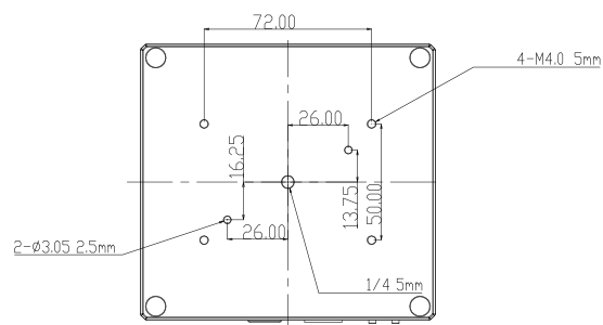
底视图
