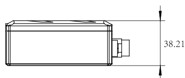
侧视图
