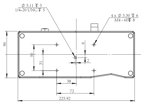
底视图
