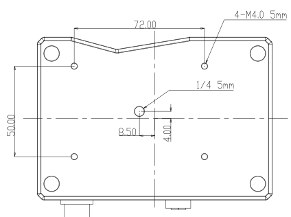
底视图
