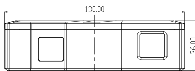
正视图
