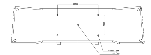
底视图
