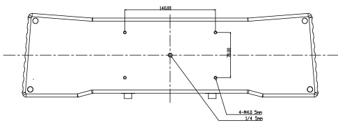
底视图
