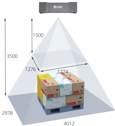
KINGFISHER-W-1201W 视野图（mm）
