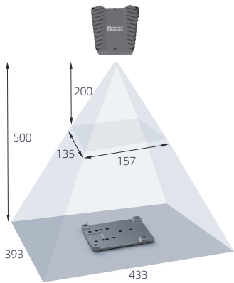
KINGFISHER-S-601 视野图（mm）
