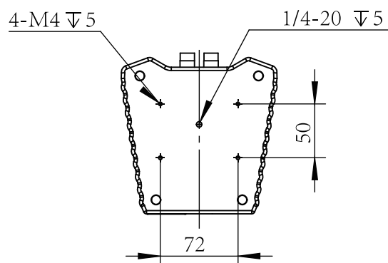
底视图
