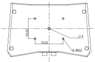
底视图
