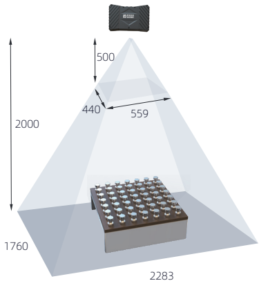
KINGFISHER-S-1201W 视野图（mm）
